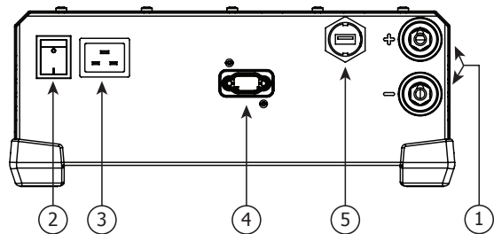
GYSFLASH 121.12 CNT
